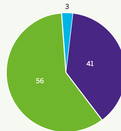
Scope 1,2,3. 2019 %
